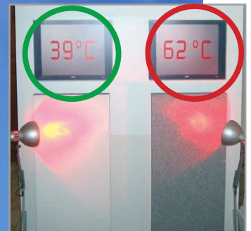
Aufheizvergleich weißer und grauer Oberflächen, bei gleicher Sonnenbestrahlung.
